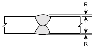
(D) ACCEPTABLE PROFILE: DOUBLE GROOVE WELD IN BUTT JOINT
